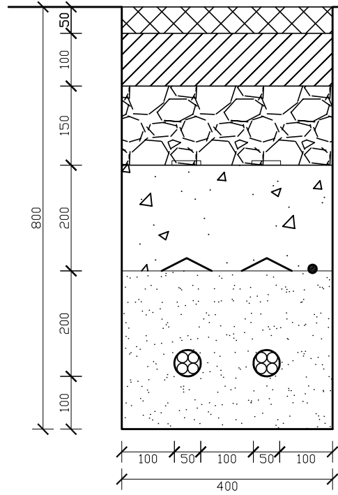
PRESJEK KB ROVA ZA POLAGANJE 2 KB 1kV U ZEMLJANOM TERENU
