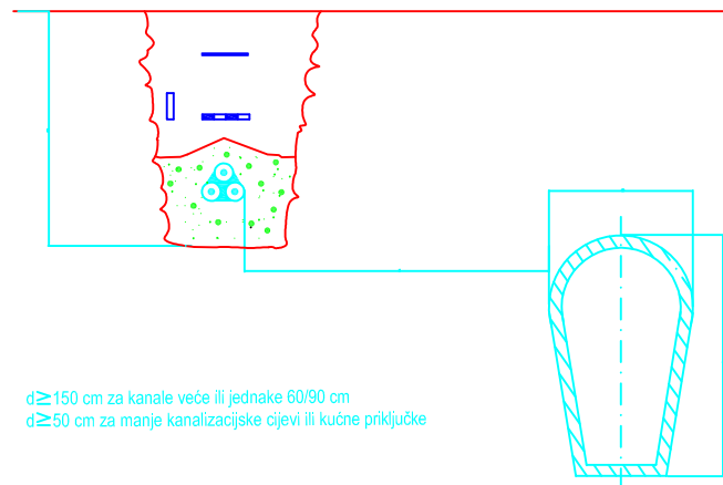
PARALELNO VODENJE I Približavanje KABELA I KANALIZACIJE
