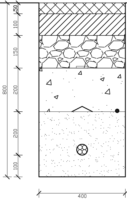
PRESJEK KB ROVA ZA POLAGANJE 1 KB 1kV U ZEMLJANOM TERENU
