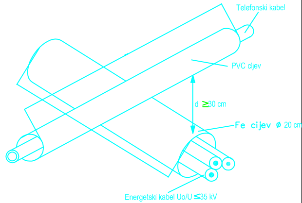
KRIŽANJE KABELA I TELEFONSKIH INSTALACIJA - SA ZAŠTITOM
